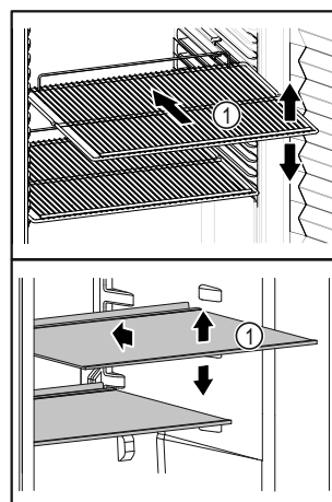
Fig. 18 Représentation à titre d'exemple
