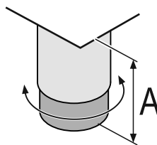
Fig. 8 Le pied réglable est réglable de A = 115 \text{ mm} ( 4 \frac{1}{2} \text{ in} ) à 175 \text{ mm} ( 6 \frac{7}{8} \text{ in} ).
