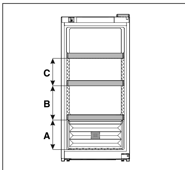
Fig. 6 Écarts entre les grilles de support
