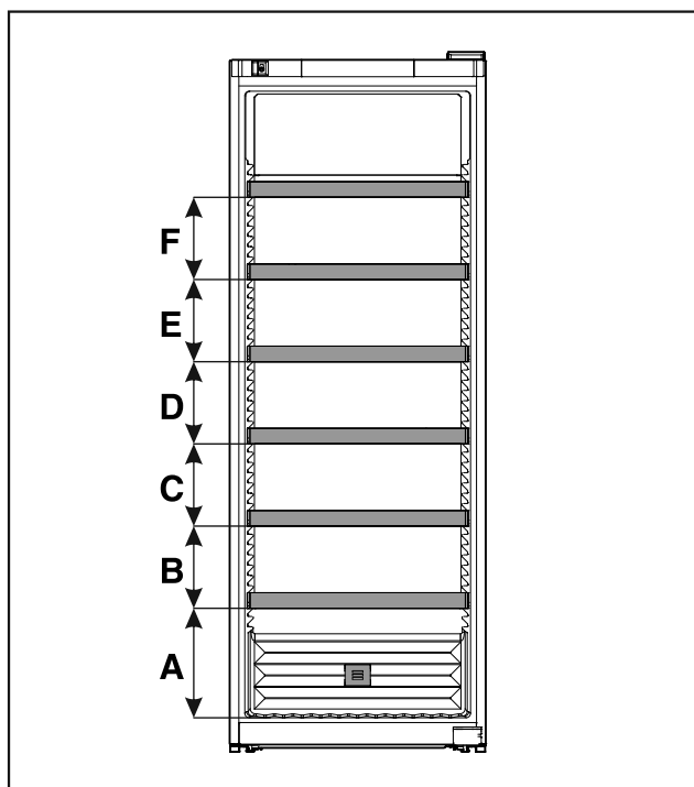
Fig. 16 Écarts entre les grilles de support
