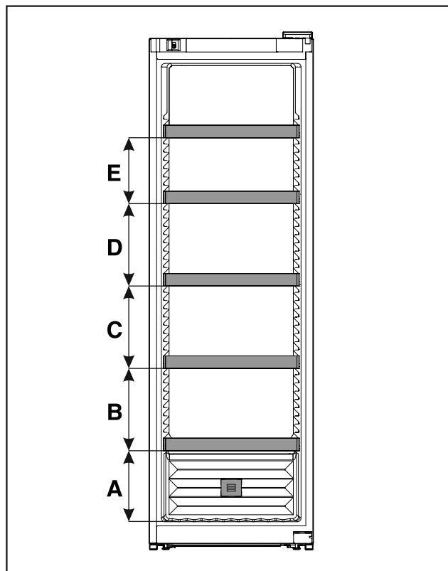
Fig. 14 Écart entre les grilles de support
