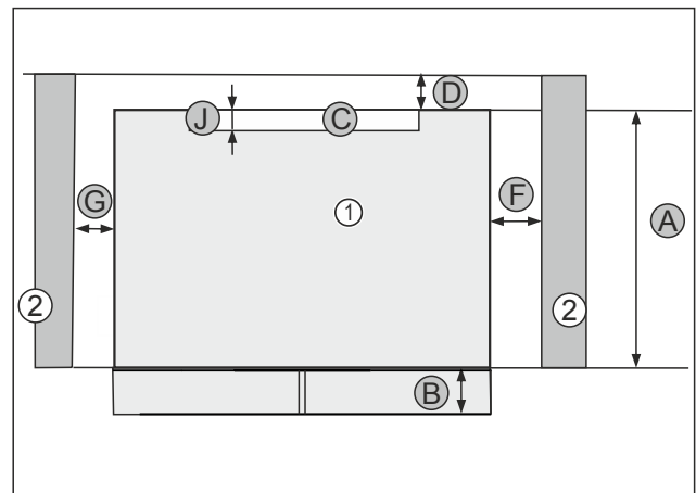
Fig. 7 Draufsicht
