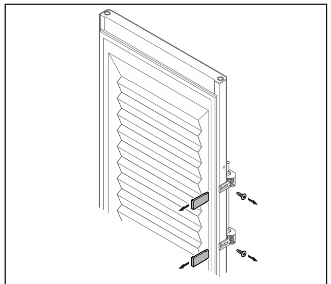
Fig. 21 Geschäumte Tür
