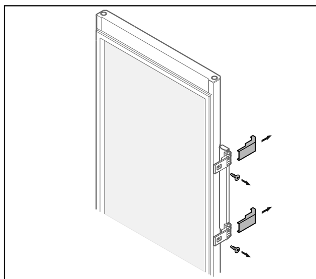
Fig. 22 Puerta de vidrio*
