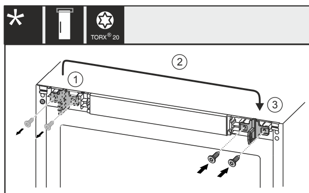
Fig. 26 con serratura elettrica*
