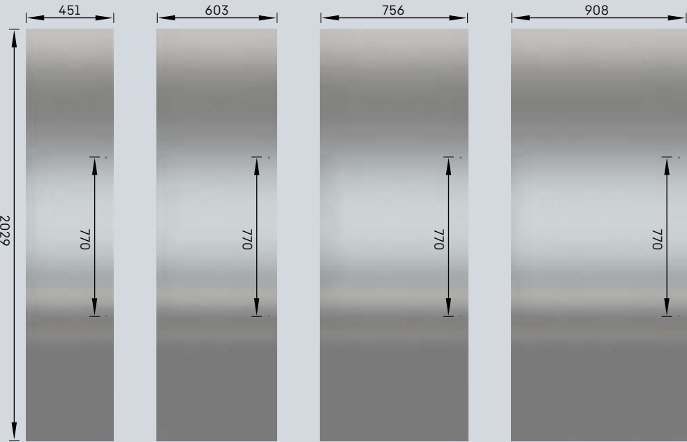
Chladničky a mrazničky
