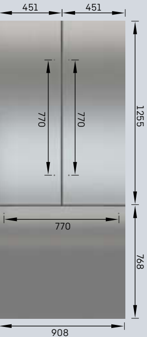
FrenchDoor (3dílná sada)
