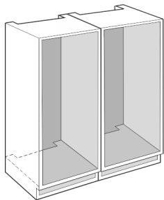
Fig. 1 Jedes Gerät in eine separate Möbelnische einbauen.
