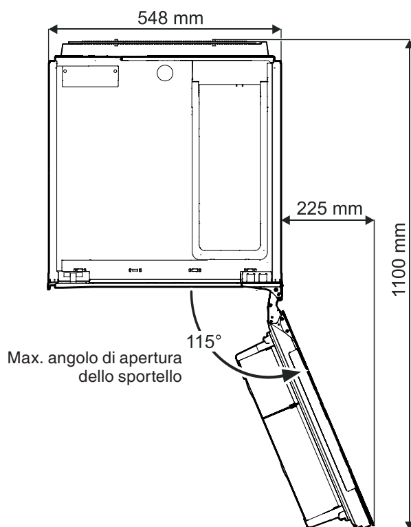
Vista dall'alto
