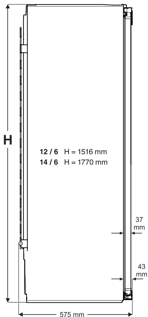
Vista laterale
