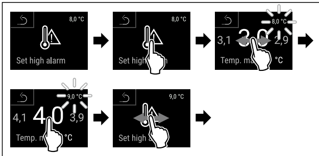
Fig. 207 Beispiel für die Einstellung der Temperaturuntergrenze, basierend auf einer eingestellten Gerätetemperatur von 5 °C.
