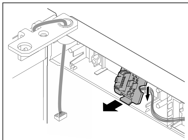
Fig. 13 Монтажную позицию держателя штекера можно повернуть на 180°.*
