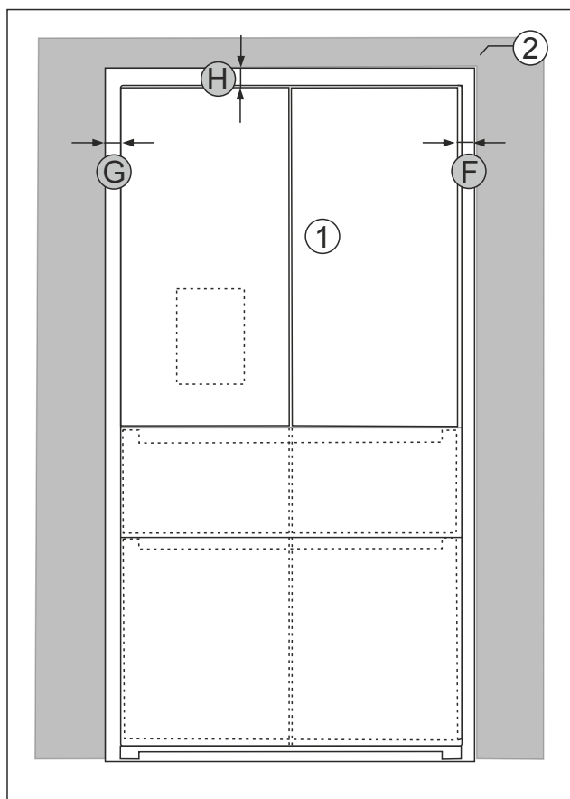
Fig. 8 Completamente circondato dal mobile da cucina (1) Apparecchio (2) Armadio della cucina (F) Distanza dal lato destro dell'apparecchio (G) Distanza dal lato sinistro dell'apparecchio (H) Distanza verso l'alto
