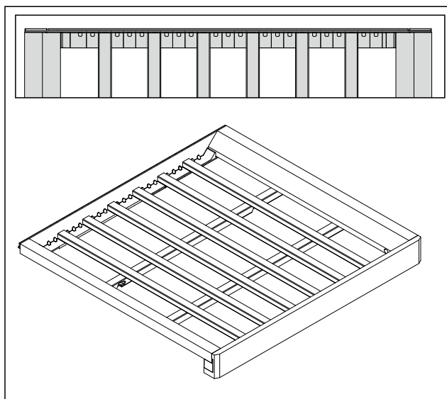
Fig. 94 最多瓶数的板条排列。
