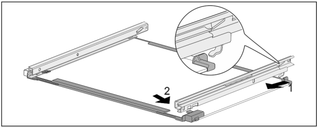
Fig. 120 带轨道的玻璃隔板 ► 轨道后部钩入。(1) ► 轨道前部卡紧。(2)
