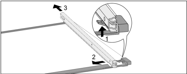
Fig. 118 带轨道的玻璃隔板 ► 向上按前端的锁定钩。(1) ► 将牵伸轨推向一侧 (2)，然后向后 (3) 推。
