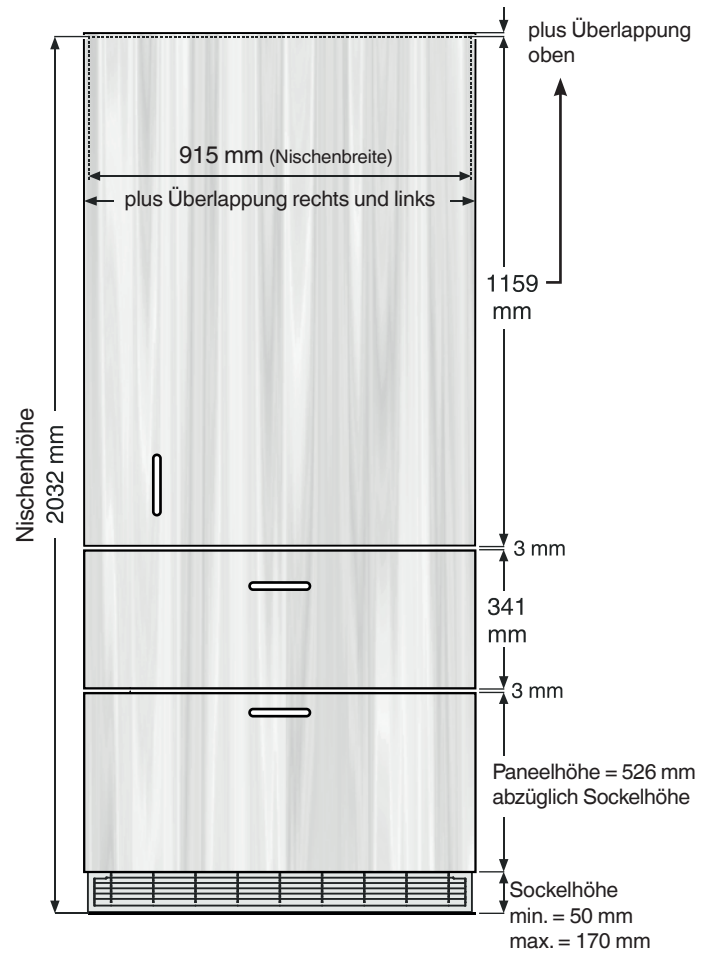
Außenliegendes Türpanel
