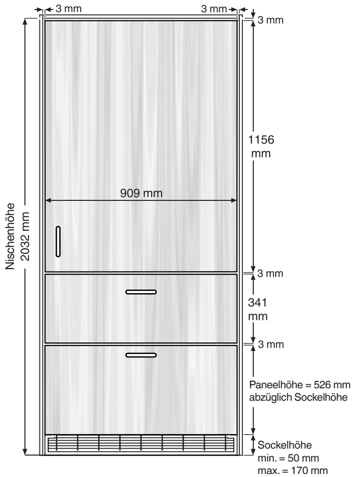
Innenliegendes Türpanel
