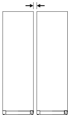
Fig. 55 Installazione Side-by-Side
