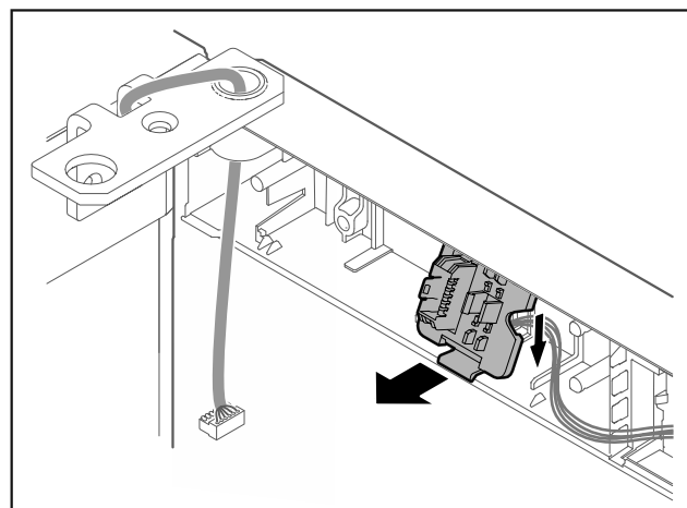
Fig. 12 La posición de instalación del soporte de la clavija de enchufe puede girarse 180°.*
