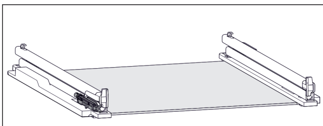
Fig. 131 Tompítóegység
