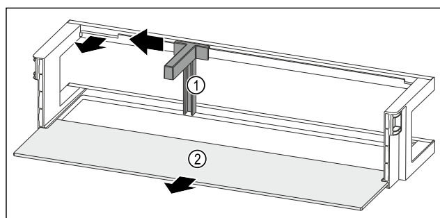
Fig. 149 带瓶托和搁板的门边存放架
