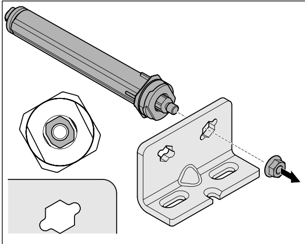
Fig. 14 Rechtsanschlag
