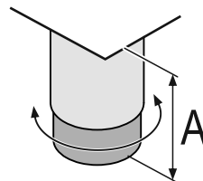
Fig. 8 Der Stellfuß ist von A = 115 \text{ mm} ( 4 \frac{1}{2} \text{ in} ) bis 175 \text{ mm} ( 6 \frac{7}{8} \text{ in} ) verstellbar.
