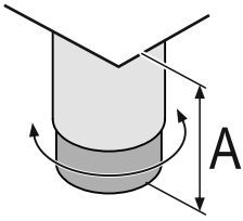
Fig. 8 Опорная ножка регулируется от A = 115 \text{ мм} ( 4 \frac{1}{2} \text{ in} ) до 175 \text{ мм} ( 6 \frac{7}{8} \text{ in} ).
