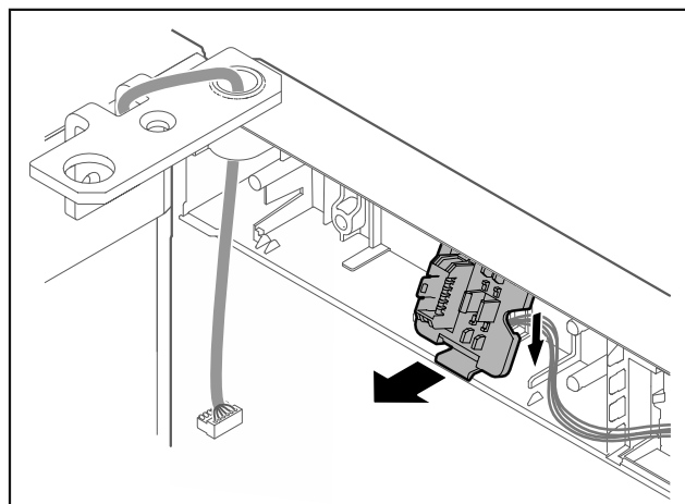
Fig. 9 Монтажную позицию держателя штекера можно повернуть на 180°.*
