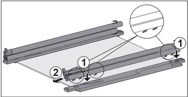
Fig. 137 带轨道和固定件的玻璃隔板
