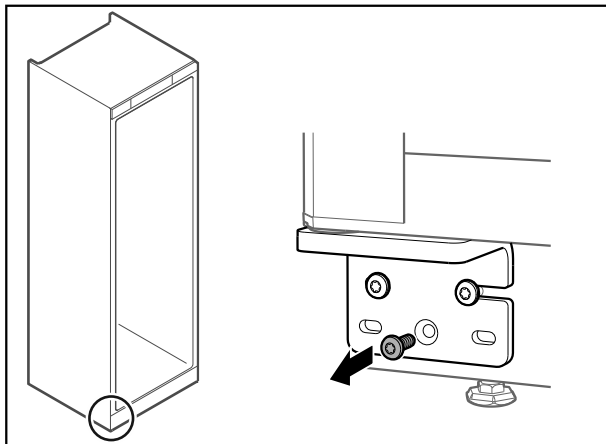
Fig. 62 Congélateur
