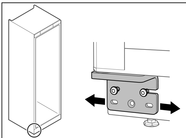
Fig. 63 Congélateur
