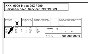
Fig. 3 Plaque signalétique
