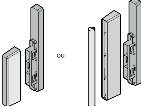
Séparateur pour le canal de ventilation au niveau du socle
