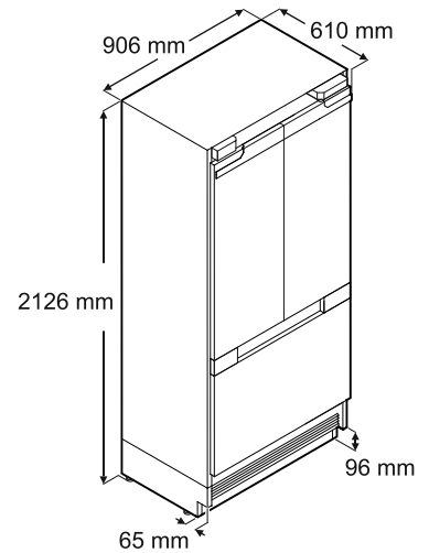
ECBN 9673 / ECBN.. 9972
