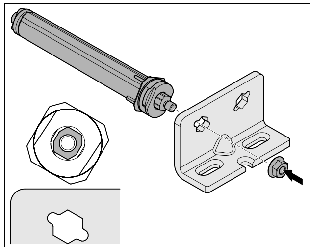
Fig. 24 Montaje de las bisagras a la izquierda
