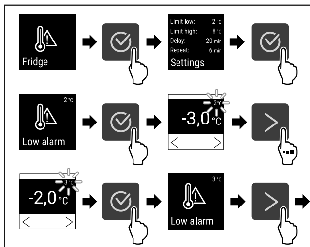
Fig. 161 Ejemplo de ajuste del límite inferior de temperatura basado en una temperatura de electrodoméstico ajustada de 5 °C.
