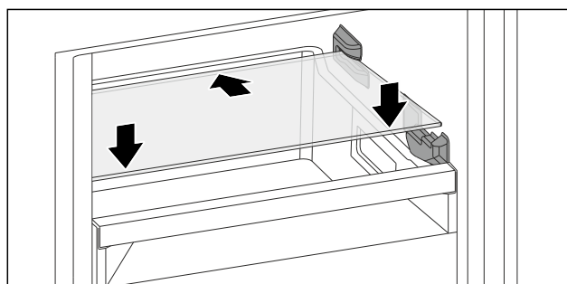
Fig. 110 玻璃隔板安装示意图
