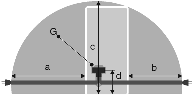
Fig. 4 制冷/冷冻组合/冰柜/全空间 BioFresh 冰箱 (a) 电源连接线最大可用的长度 (d) 冰箱插头到地面的距离 (b) 电源连接线最大可用的长度 (G) 冰箱插头 (c) 电源连接线最大可用的垂直长度
