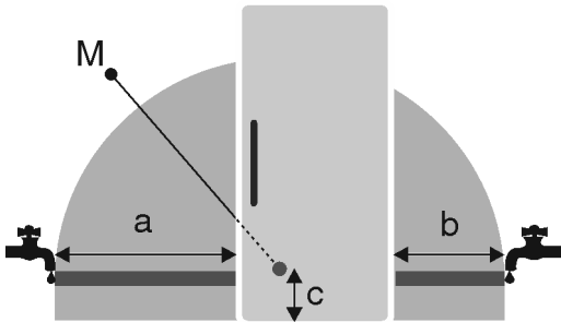
Fig. 5 (a) 最大可用的软管长度 (c) 电磁阀到底部的距离 (b) 最大可用的软管长度 (M) 电磁阀
