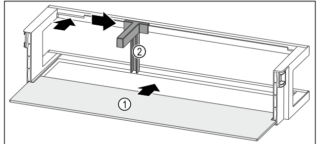
Fig. 136 Balconcino controporta con ripiano
