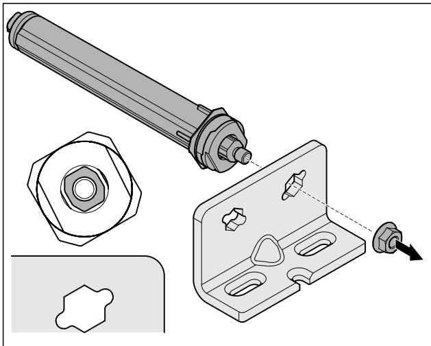
Fig. 24 Rechtsanschlag
