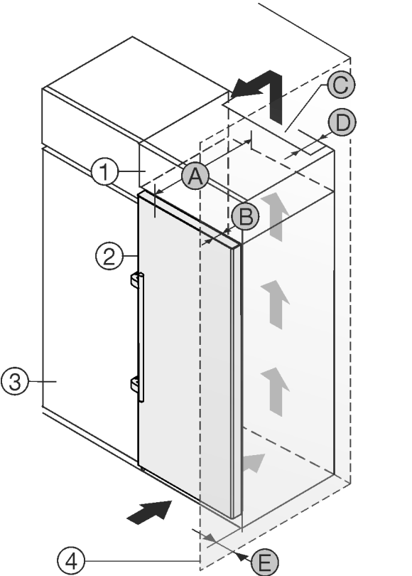
Fig. 25 (1) 附加柜 (2) 冰箱 (3) 餐具柜 (4) 墙壁 (A) 冰箱深度 (B) 门深度 (C) 通风横截面 (D) 冰箱背面间距 (E) 到冰箱侧面的间距
