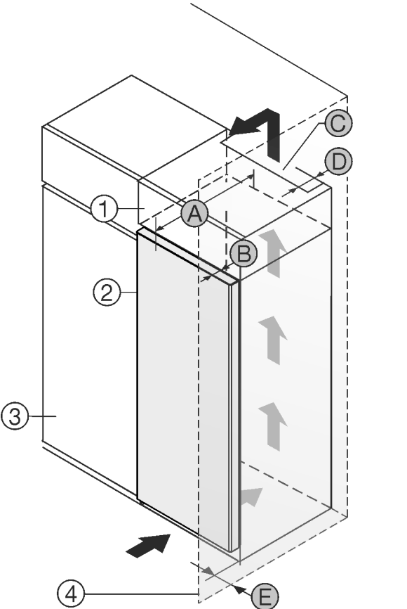
Fig. 24 (1) 附加柜 (2) 冰箱 (3) 餐具柜 (4) 墙壁 (A) 冰箱深度 (B) 门深度 (C) 通风横截面 (D) 冰箱背面间距 (E) 到冰箱侧面的间距
