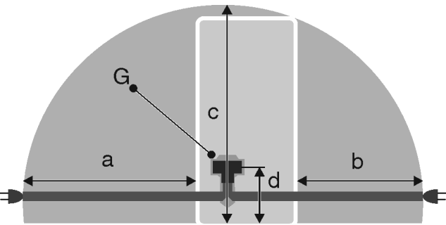
Fig. 3 制冷/冷冻组合/冰柜/全空间BioFresh 冰箱 (a) 电源连接线最大可用的长度 (b) 电源连接线最大可用的长度 (c) 电源连接线最大可用的垂直长度 (d) 冰箱插头到地面的距离 (G) 冰箱插头
