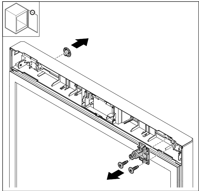
Fig. 32 Beispielhafte Darstellung: Geschäumte Tür
