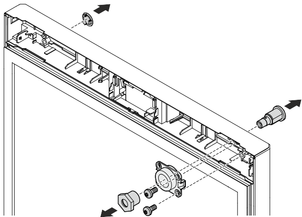
Fig. 33 Beispielhafte Darstellung: Glastür
