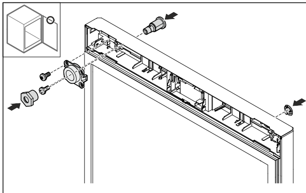
Fig. 35 Beispielhafte Darstellung: Glastür
