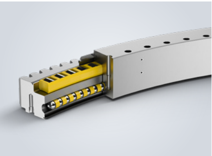
Kombinierte Rollen-Kugel-Drehverbindung Außen-/innen-/unverzahnt
