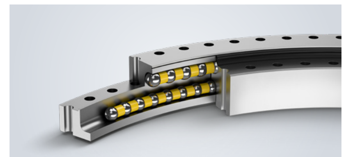
Zweireihige Kugeldrehverbindungen Zweipunktkontakt – außen-/innen-/unverzahnt
