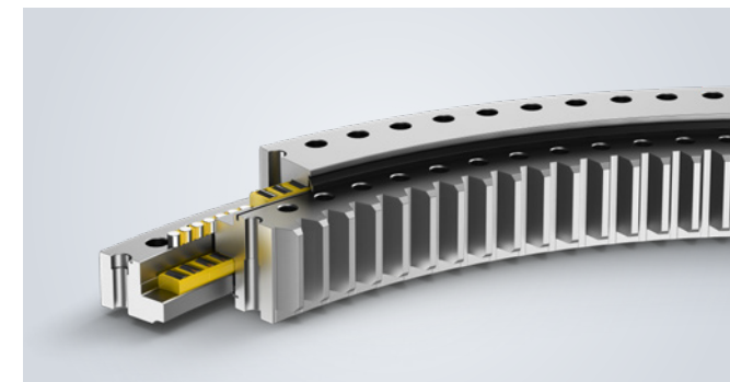
Dreireihiges Rollenlager Außen-/innen-/unverzahnt
