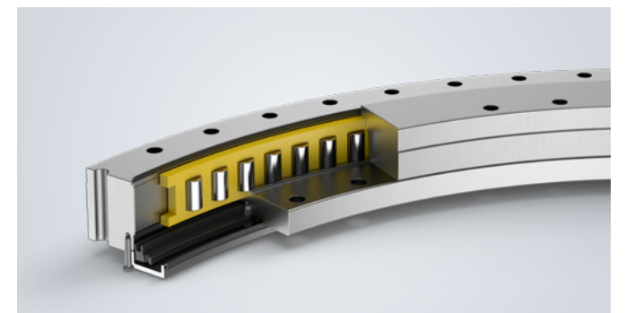
Radial-Rollenlager Außen-/innen-/unverzahnt
