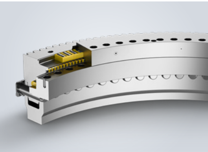
Drehverbindungen mit spezieller Anschlusskonstruktion Außen-/innen-/unverzahnt
