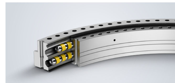
Zweireihige Vierpunktlager Doppel-Vierpunktkontakt – außen-/innen-/unverzahnt
