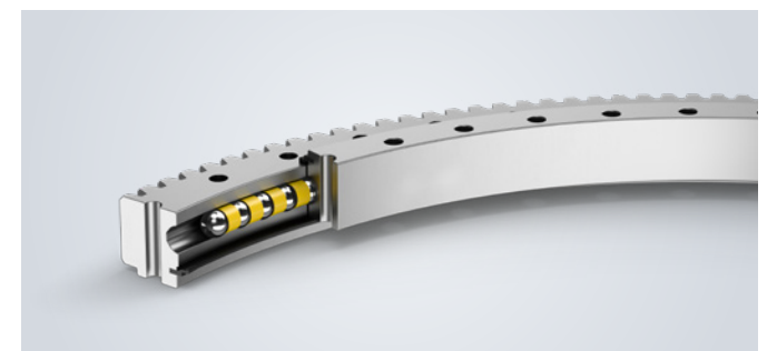
Einreihige Vierpunktlager Vierpunktkontakt – außen-/innen-/unverzahnt
