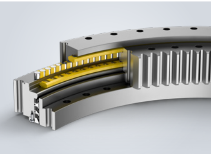
Dreireihiges Rollenlager Mit Spezialdichtungen – außen- oder innenverzahnt
