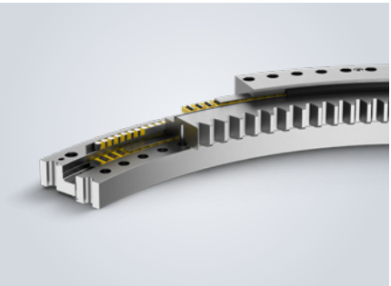
Segmentiertes Lager Alle Durchmesserbereiche – außen-/innen-/unverzahnt
