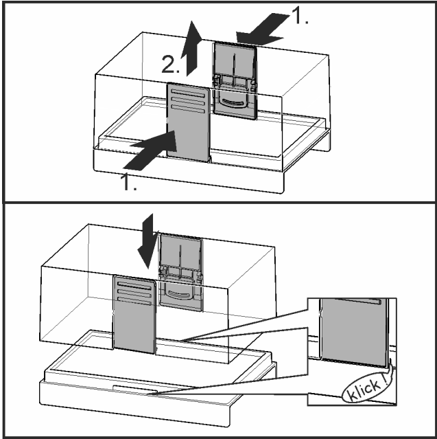
Fig. 44 拆卸黄油盒
