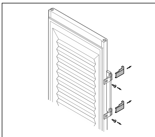
Fig. 22 Zapěněná dvířka
