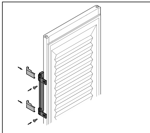
Fig. 24 Zapěněná dvířka
