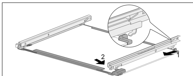
Fig. 215 Tablette en verre avec rails
