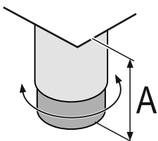
Fig. 51 La pata de ajuste se puede regular desde A = 115 \text{ mm} (4 1/2 in) a 175 \text{ mm} (6 7/8 in).*
