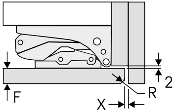
Fig. 65 Fugenspalt mit anschließender Möbelwanne (F) Frontdicke (X) Fugenspalt min. (R) Eckradius Möbelfront
