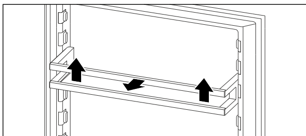
Fig. 48 Beispielhafte Darstellung ► Türabsteller nach oben schieben. ► Türabsteller nach vorne ziehen.
