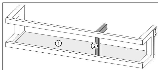
Fig. 147 Beispielhafte Darstellung Türabsteller (1) Abstellfläche
