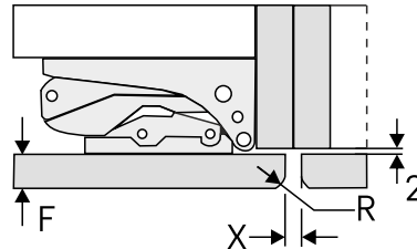
Fig. 67 Fugenspalt mit anschließender Möbeltür
