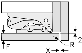
Fig. 66 Fugenspalt mit anschließender Möbelwanne
