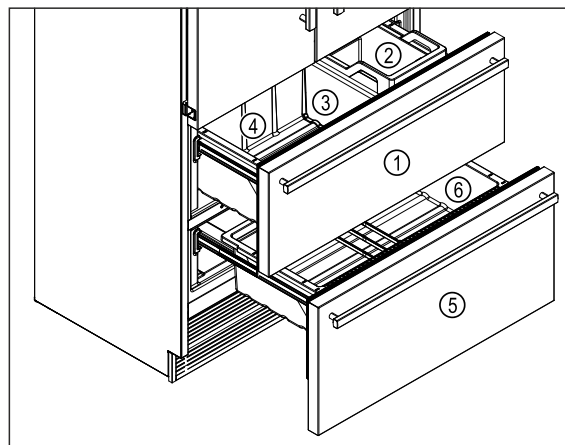
Fig. 73 Auszugswagen Gefrierteil
