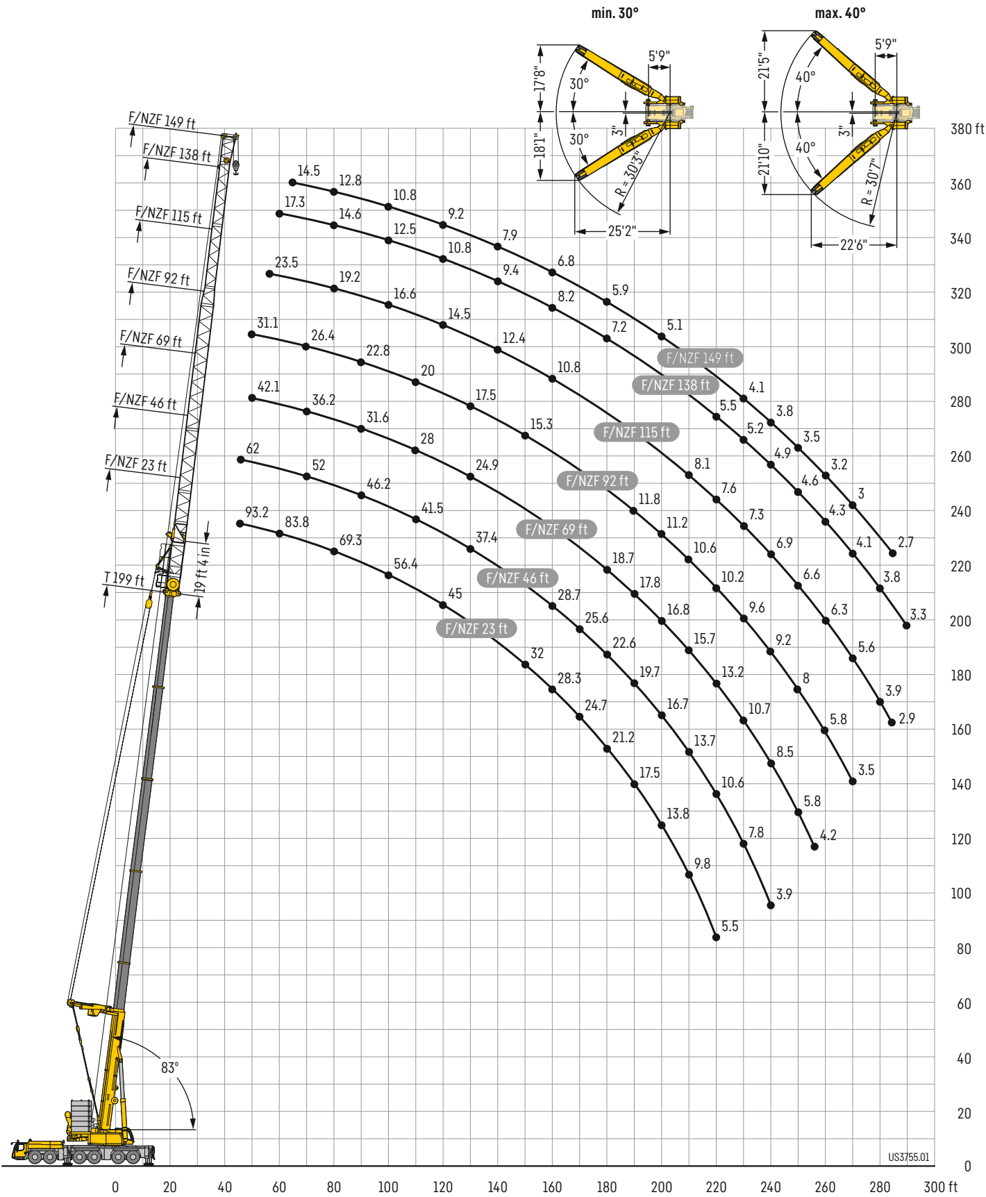
Angle of the Y-suspension between 30° and 40° depending on the extension condition of the individual telescopic sections Angle du haubannage Y entre 30° et 40°, en fonction de l'état de sortie des différents éléments télescopiques
