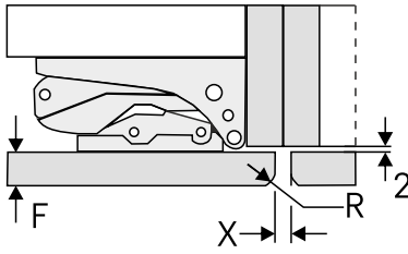
Fig. 101 Fessura con porta del mobile adiacente (F) Spessore parte frontale (X) Fessura min. (R) Raggio angolare parte frontale del mobile
