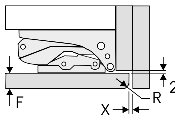
Fig. 100 Fessura con pannello laterale del mobile adiacente
