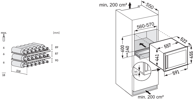
安装示意图
