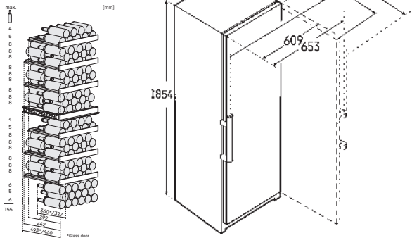
安装示意图
