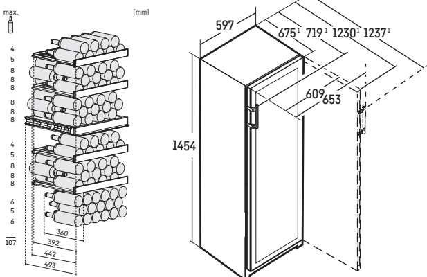
安装示意图
