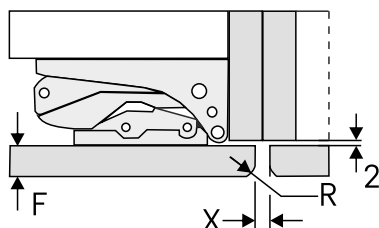
Fig. 96 Fessura con porta del mobile adiacente
