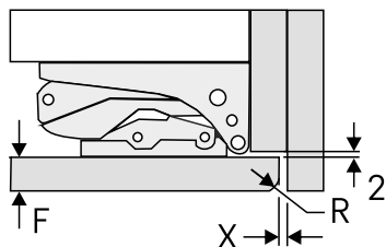
Fig. 95 Fessura con pannello laterale del mobile adiacente
