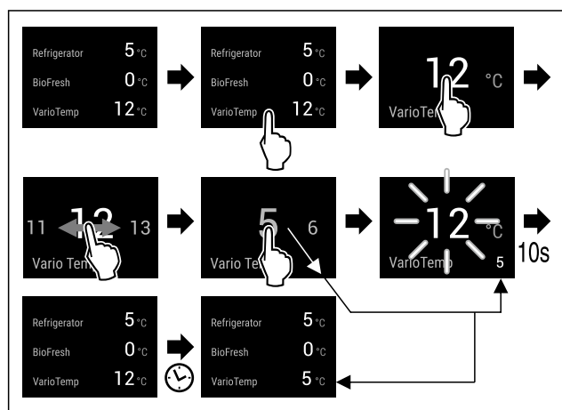
Fig. 117 Beispielhafte Darstellung: VarioTemp von 12 °C auf 5 °C für eine Kühl-Gefrier-Kombination mit BioFresh ändern.
