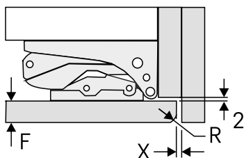
Fig. 93 Fugenspalt mit anschließender Möbelwanne
