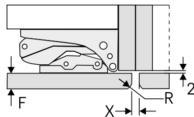
Fig. 94 Fugenspalt mit anschließender Möbeltür
