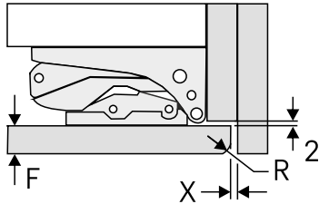
Fig. 67 Fugenspalt mit anschließender Möbelwanne (F) Frontdicke (X) Fugenspalt min. (R) Eckradius Möbelwanne
